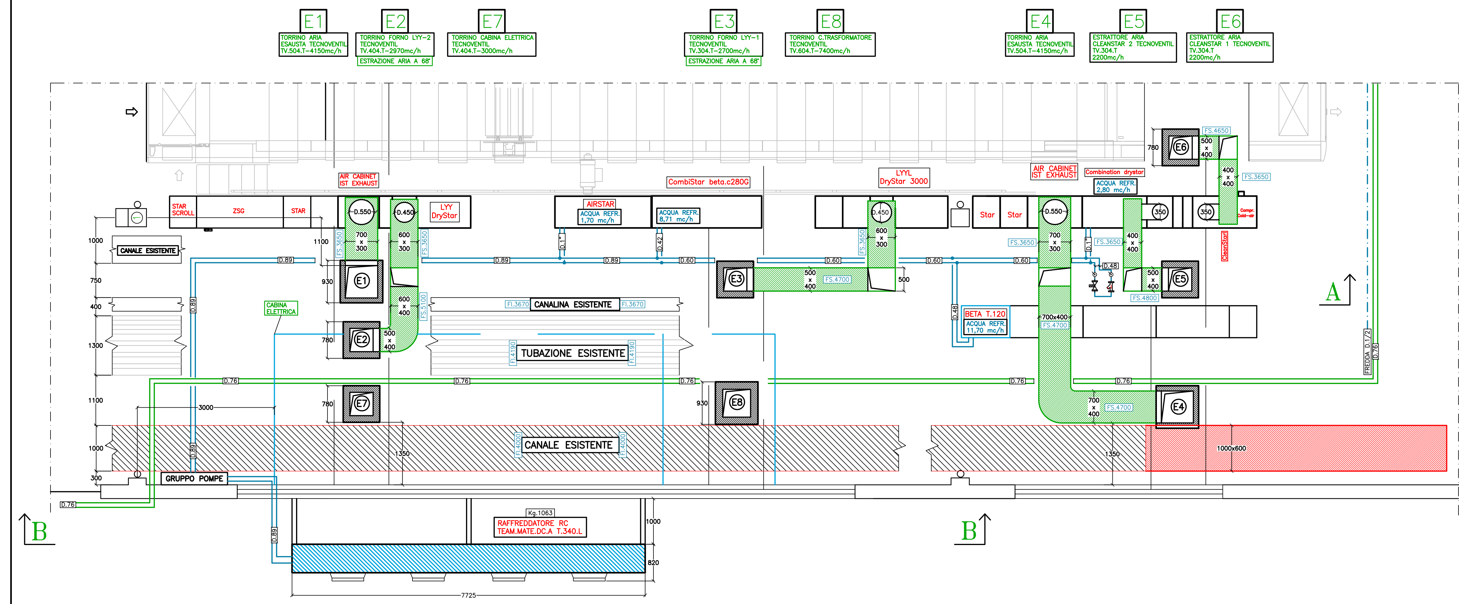
PIANTA
